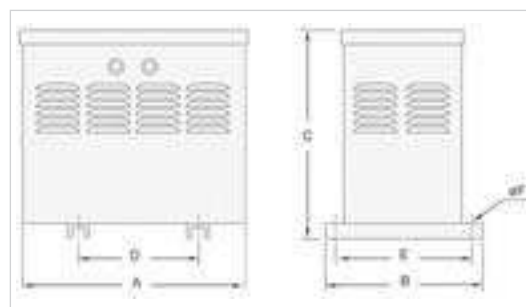
Dimensions TRT 30 IP23
