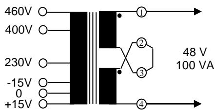
CONEXIÓN SERIE SERIAL CONNECTION
