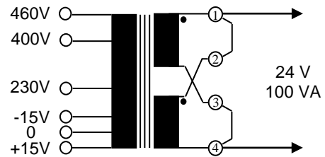
CONEXIÓN PARALELO PARALLEL CONNECTION
