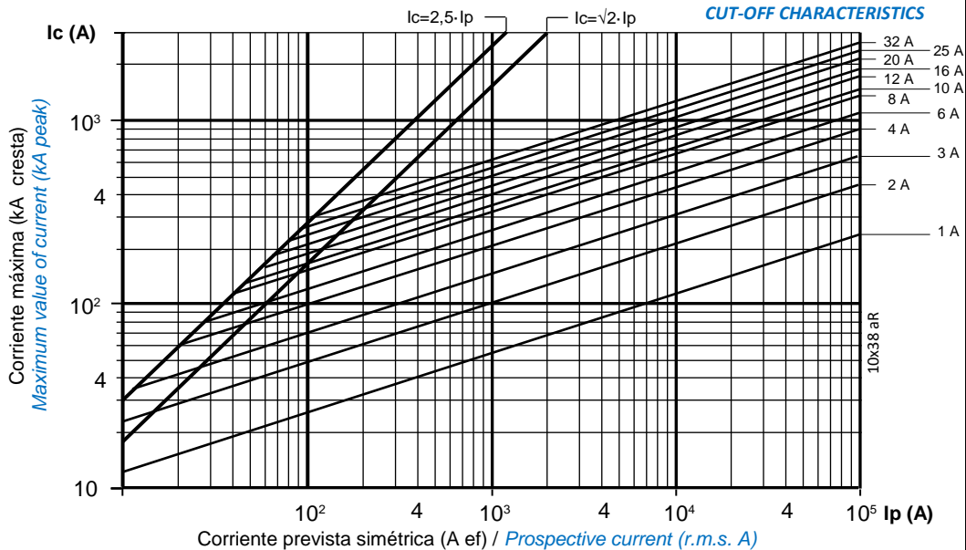
CARACTERÍSTICAS DE LIMITACIÓN CUT-OFF CHARACTERISTICS
